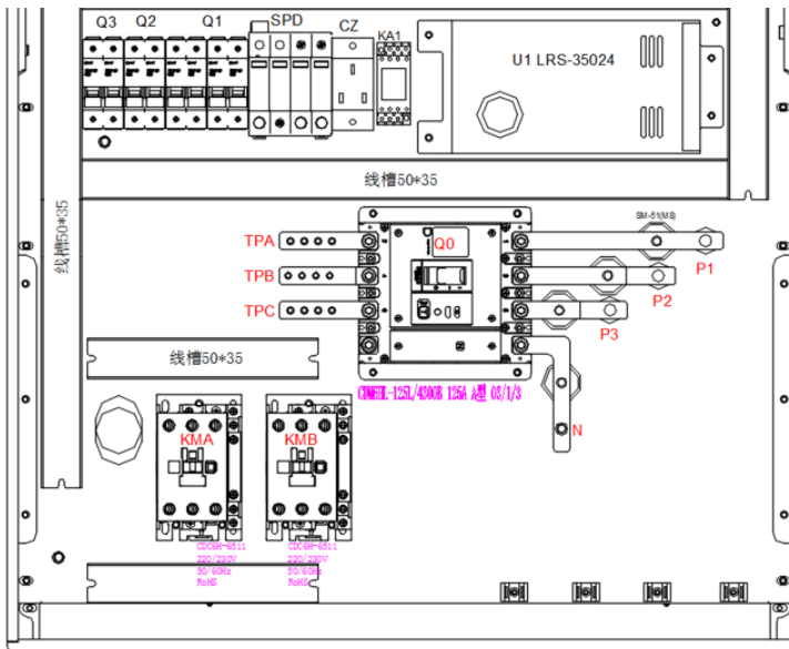
Imagem 11 – Visão interna do circuito de entrada do carregador DC Nansen
